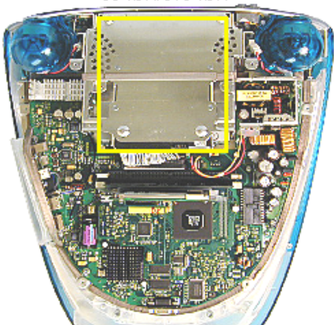
CD-ROM/DVD ROM
